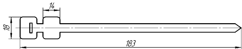
Рис. 3.3.7 Держатель ДМОУ-С пр.
