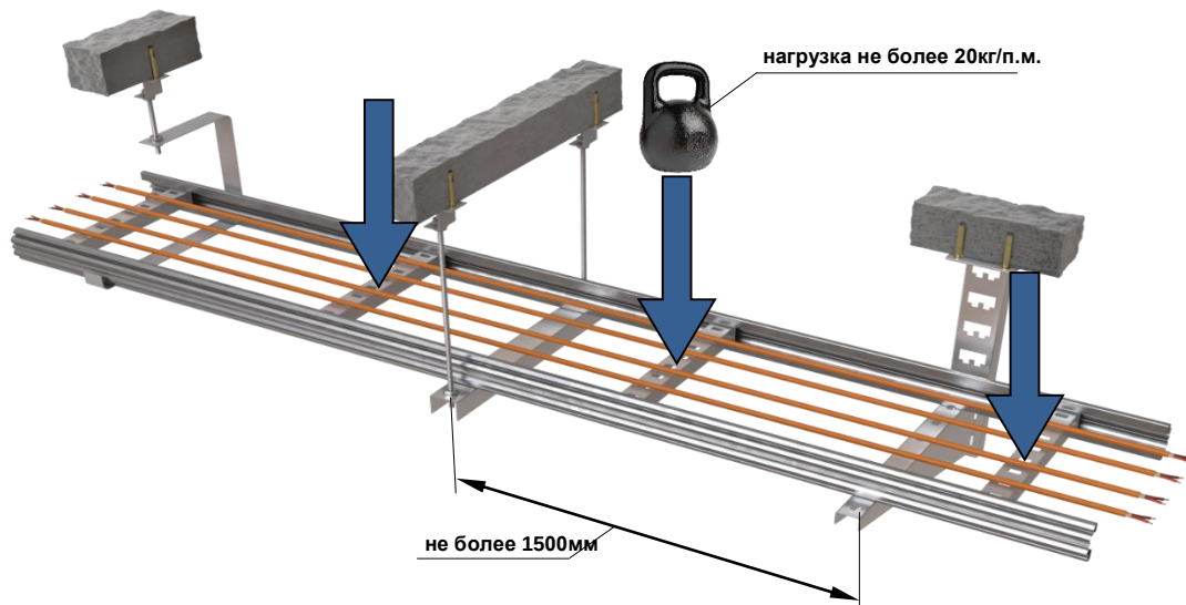
Рис. 2.11.1 Схема монтажа ОКЛ «ПжТехКабель РТК-Line-ЛМЛО»
