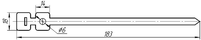
Рис. 3.3.6 Держатель ДМОУ-С
