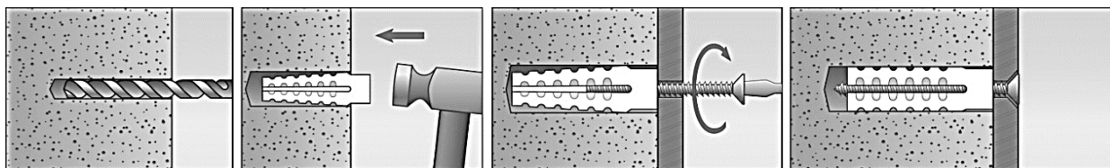
Рис. 2.2.8 Последовательность монтажа дюбеля металлического с саморезом
