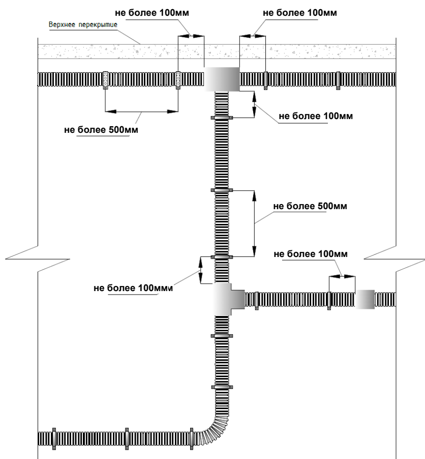
Рис. 2.7.1 Схема монтажа ОКЛ «ПожТехКабель РТК-Line-РМ» и «ПожТехКабель РТК-Line-РМП»
