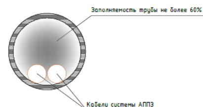
Расположение кабеля в металлорукаве с х/б уплотнением
