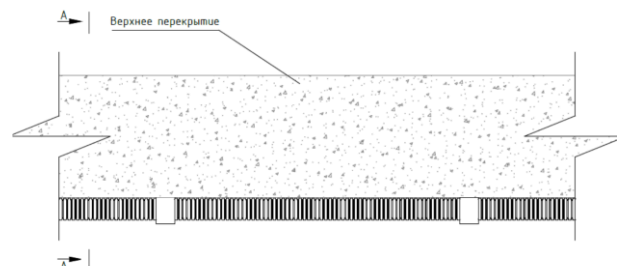
Схема прокладки кабелей в металлорукаве с х/б уплотнением с креплением на горизонтальной плоскости
