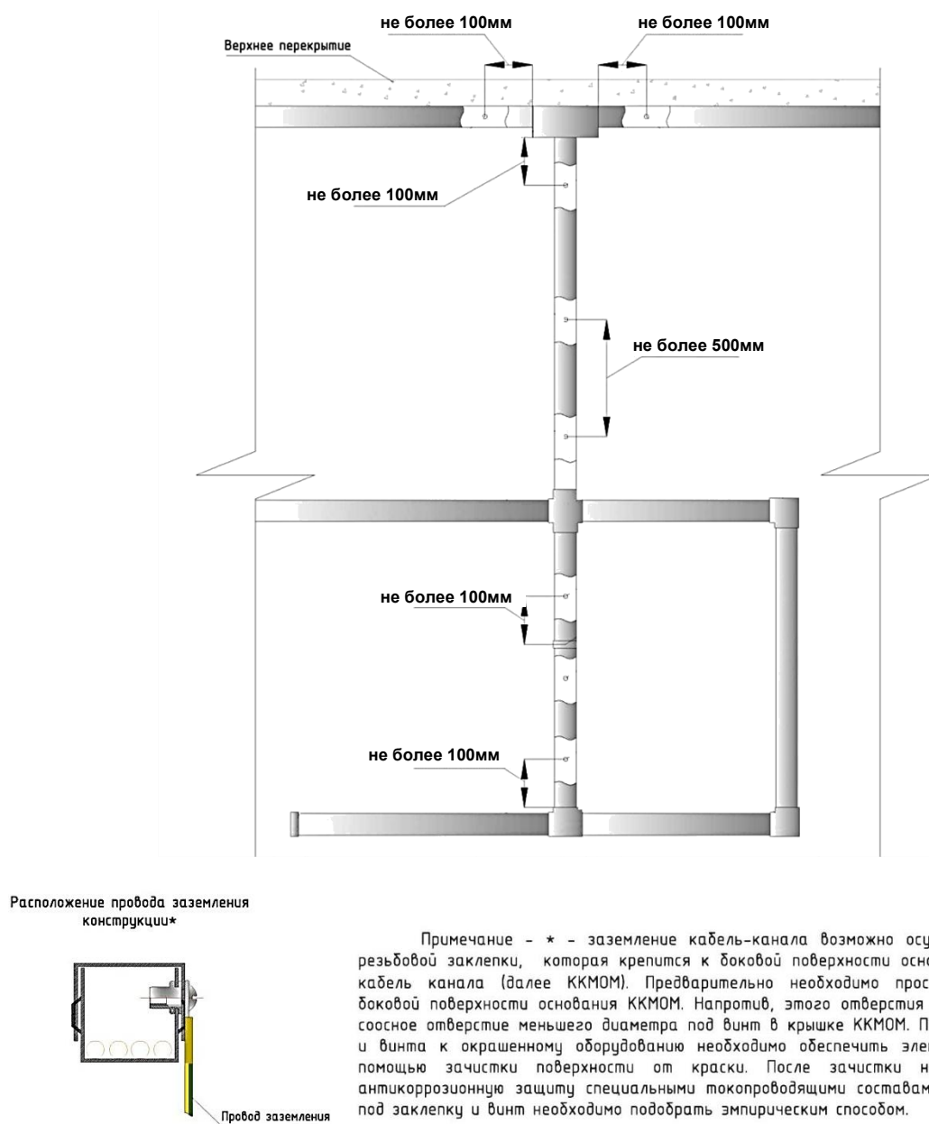
Рис.2.4.1 Схема монтажа «ПожТехКабель РТК-Line-ККМОМ» на вертикальной плоскости с учетом организации заземления
